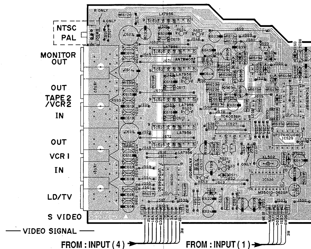
RX-V1070/V870 DSP P. C. B. ( 3 )
