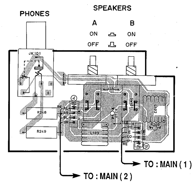
RX-V1070 MAIN P. C. B. ( 4 )
