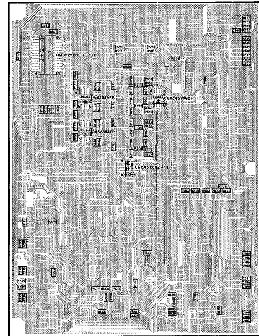
RX-V1070/V870 DSP P. C. B. ( 2 )
