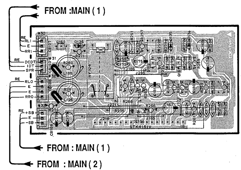
RX-V1070 MAIN P. C. B. ( 5 )
