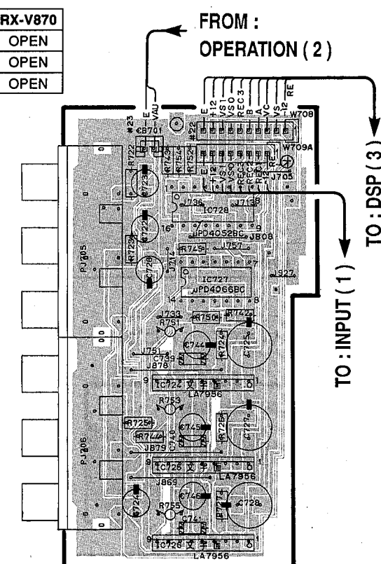
RX-V1070/V870 INPUT P. C. B. ( 4 )
