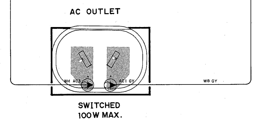
RX-V1070 MAIN P. C. B. ( 7 )
