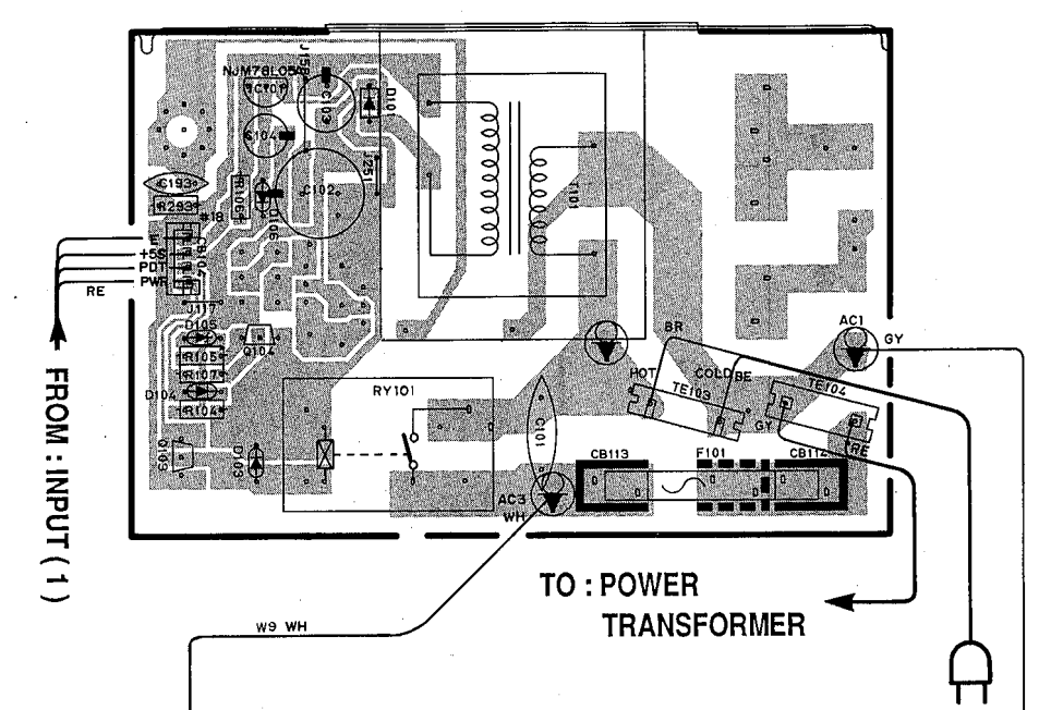
RX-V1070 MAIN P. C. B. ( 3 )
