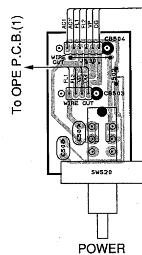
OPE P.C.B.(2)
