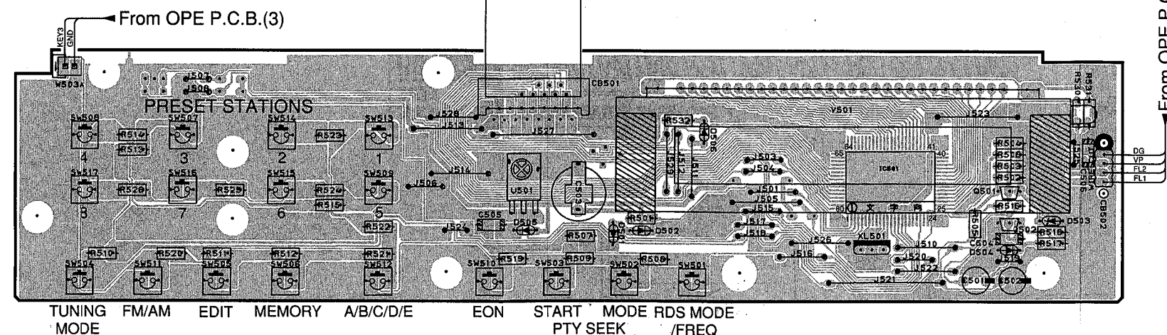
OPE P.C.B.(1)
