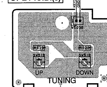
OPE P.C.B.(3)
