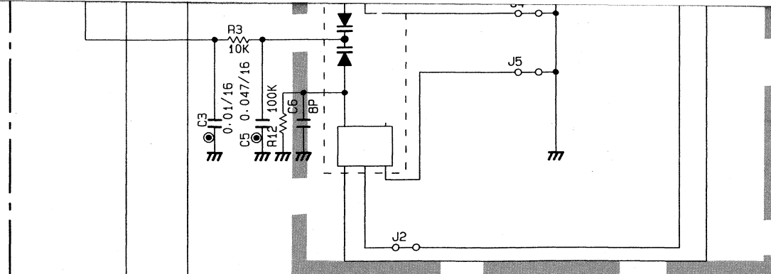
IC1 : LC72130 (PLL)
