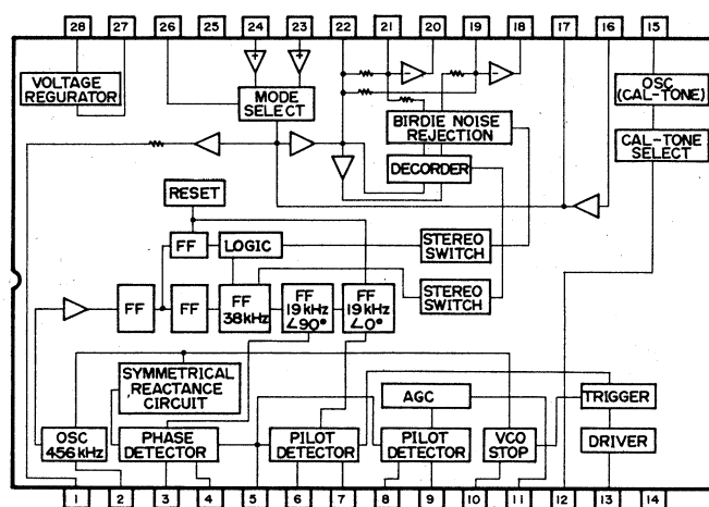
IC106: LA3450 (MPX)
