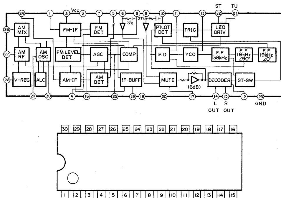
IC1 : LA1851N
