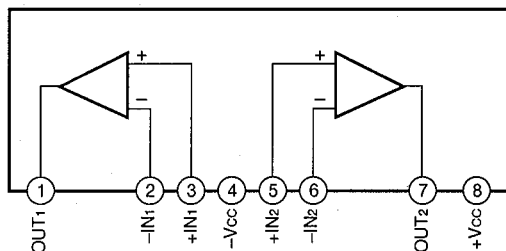
IC11 : NJM4558L Dual OP-Amp
